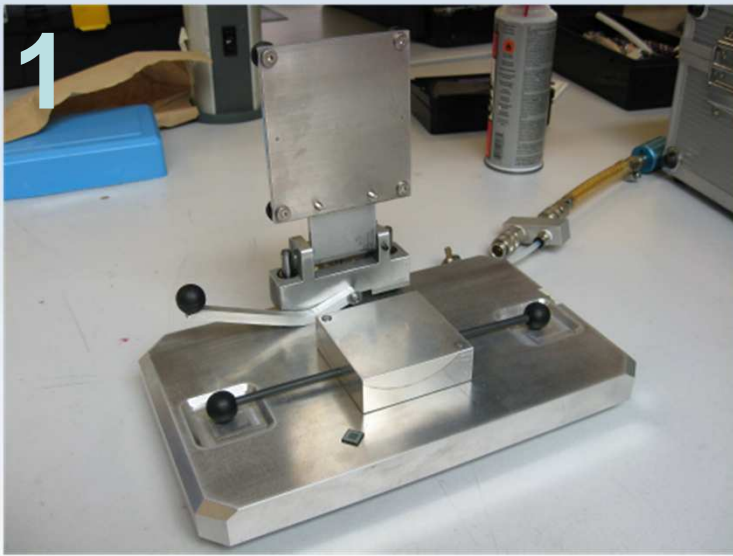
Placer le composant:
