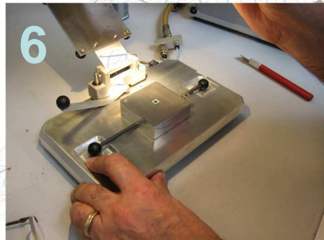
Actionner la manette de démoulage puis relever le stencil:
