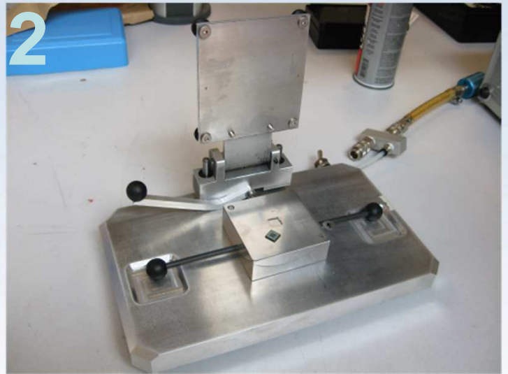
Installer le cadre de composant:
