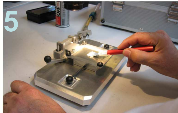
Déposer la crème à braser avec la raclette appropriée:
